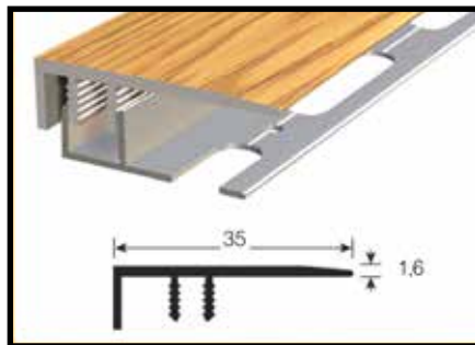
Junta Remate final Medida: 2700x35 mm
