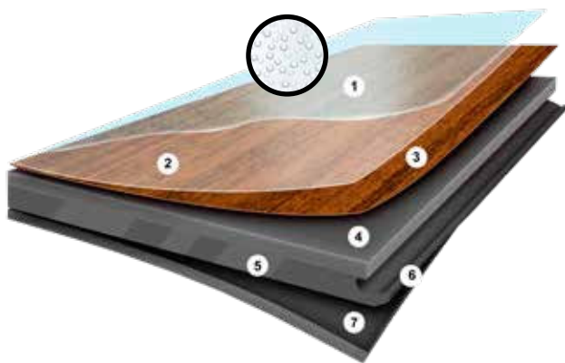
Composición de los suelos vinílicos con tecnología Isocore
