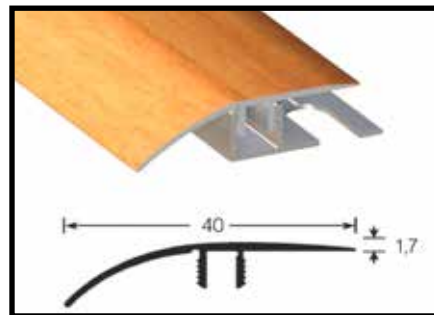
Junta de transición Medida: 900x40 mm
