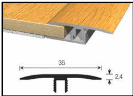
Junta de dilatación Medida: 900x35 mm
